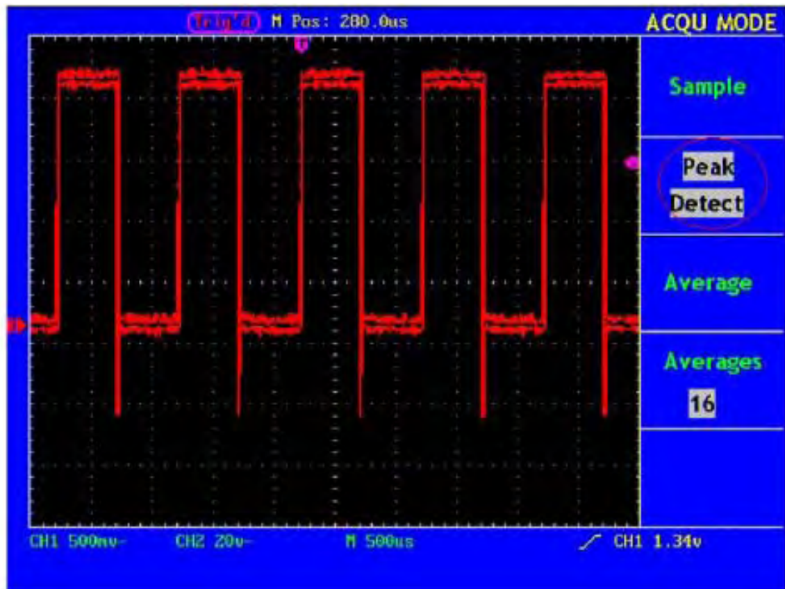
Abb. 34 Peak Detect Mode, mit deren Hilfe die Spitzen der fallenden Flanke ermittelt werden können und Rauschen festgestellt wird.
