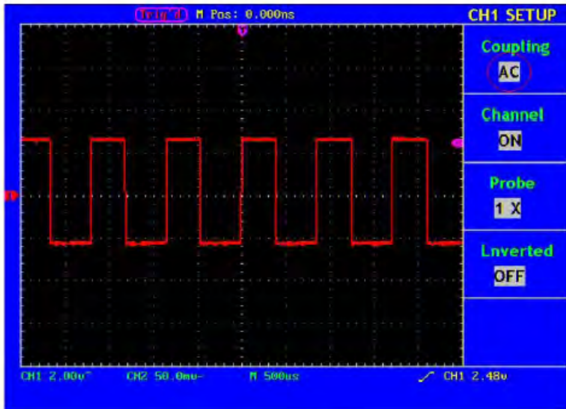
Abb.15 Kopplung Oscillogram
