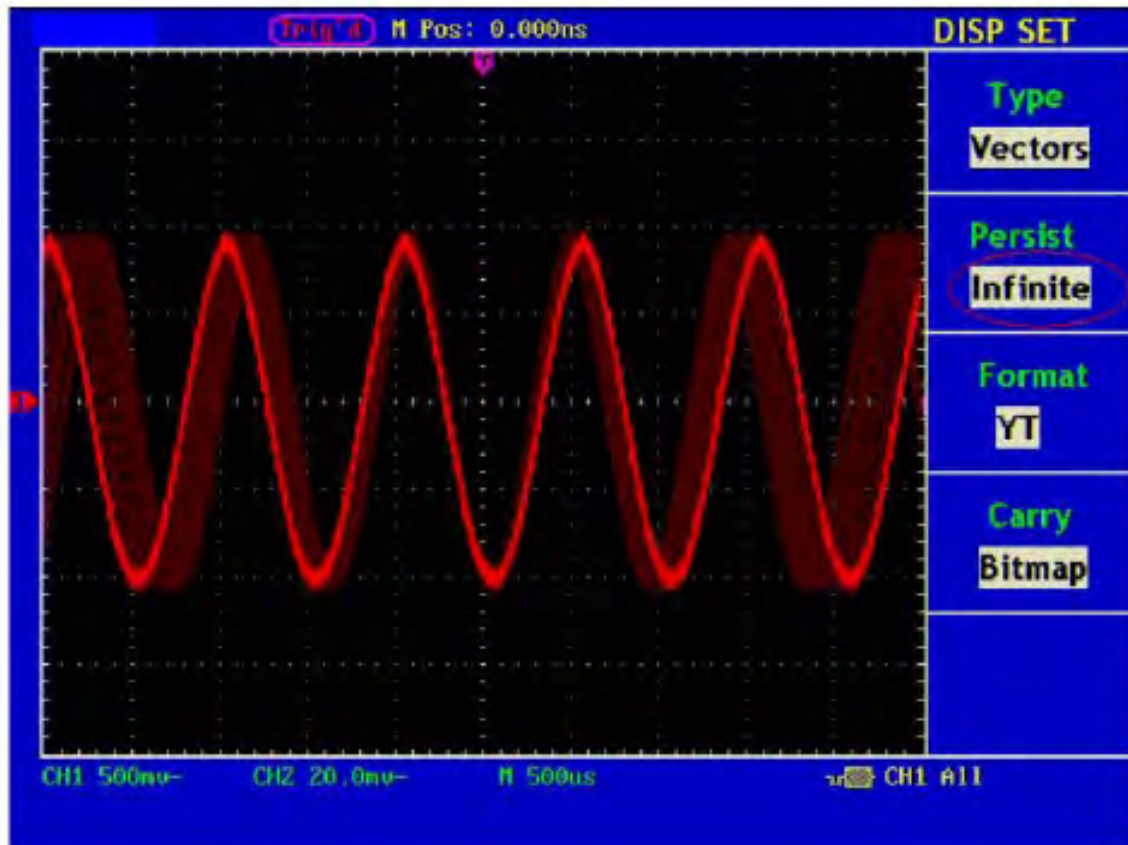
Abb. 40 Unendliche Nachleutzeit
