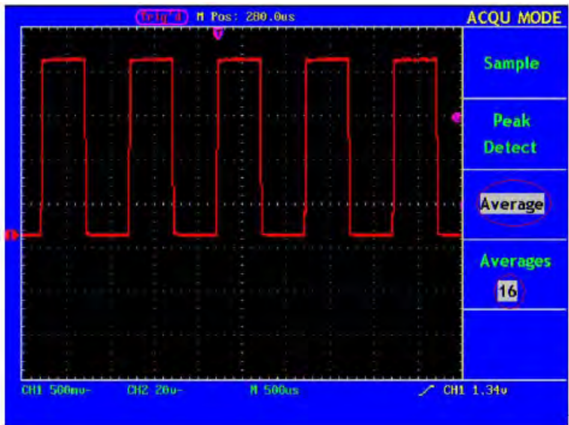
Abb. 57 Wellenform eines von Störungen befreiten Signals
