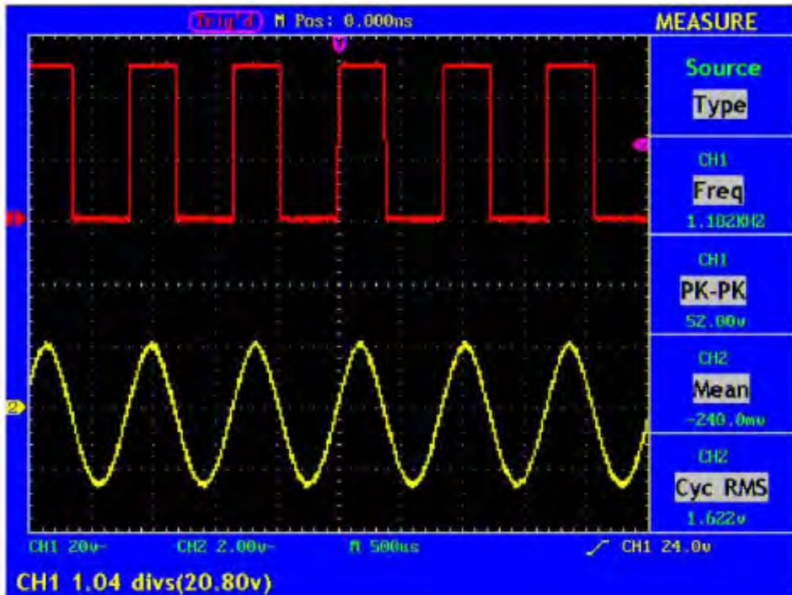
Abb. 49 automatische Messungen
