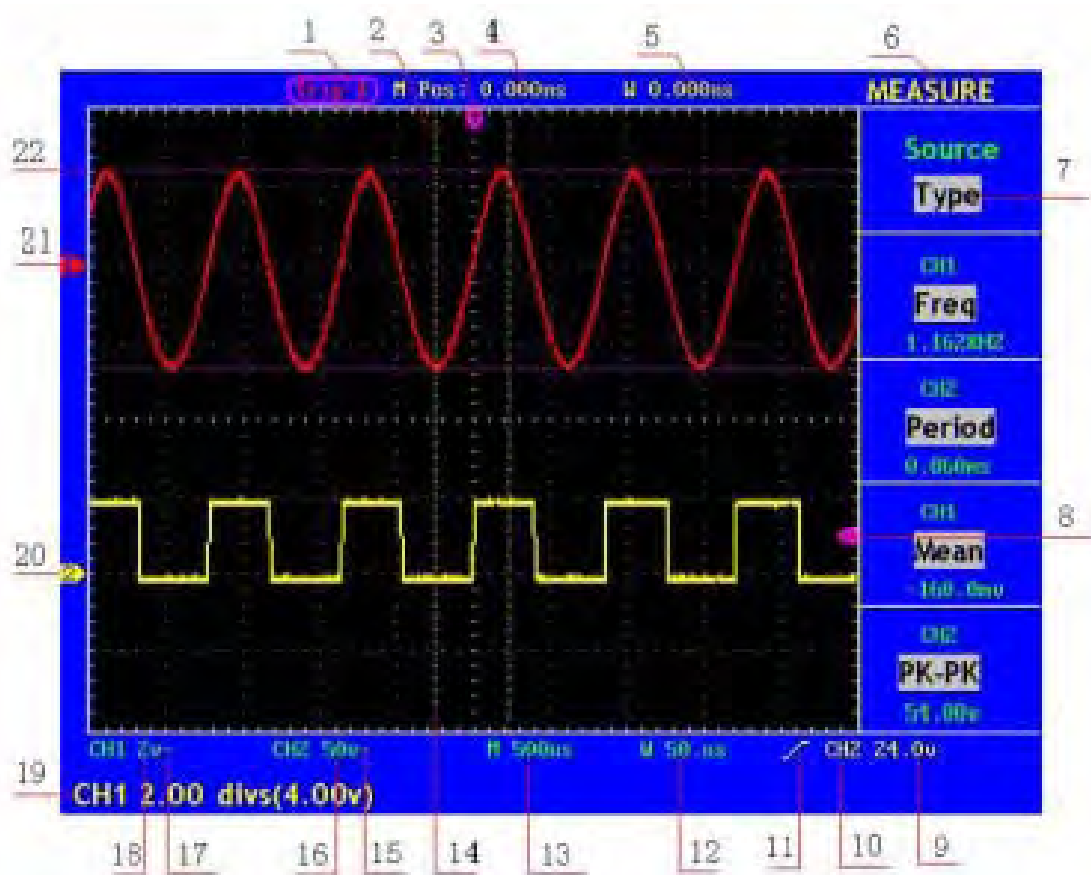
Abb. 3 Bedienoberfläche
