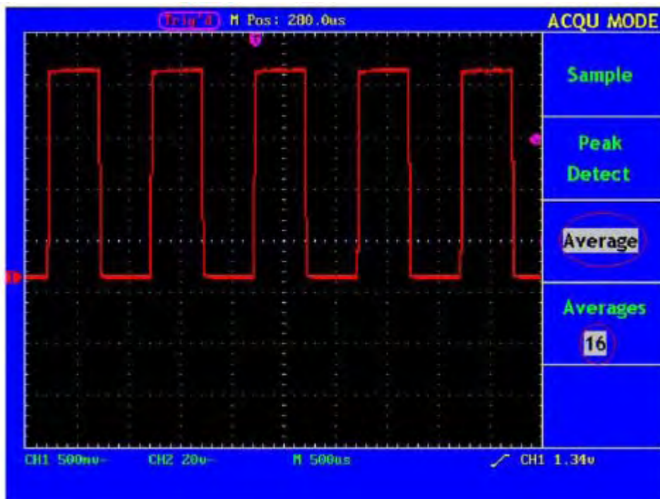
Abb. 36 die angezeigte Wellenform nachdem das Rauschen mit dem Average Mode entfernt wurde. Die Averagenummer wurde eingestellt auf 16.
