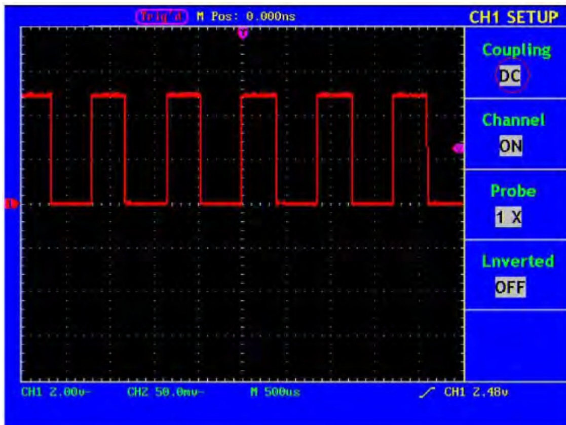
Fig. 16 DC Coupling Oscilloscope
