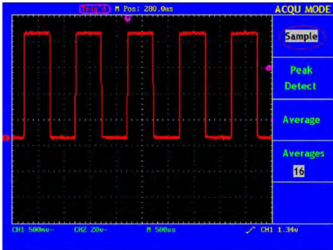
Abb. 35 übliche ACQU-Mode-Anzeige an der keine Spitzen ermittelt werden können
