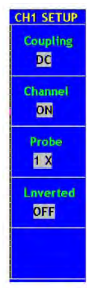
Abb. 14 Kanal-Einstellmenü
