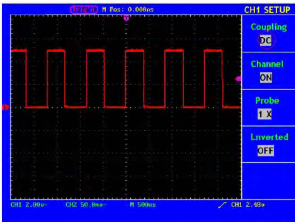
Abb.15 Kopplung Oscillogram
