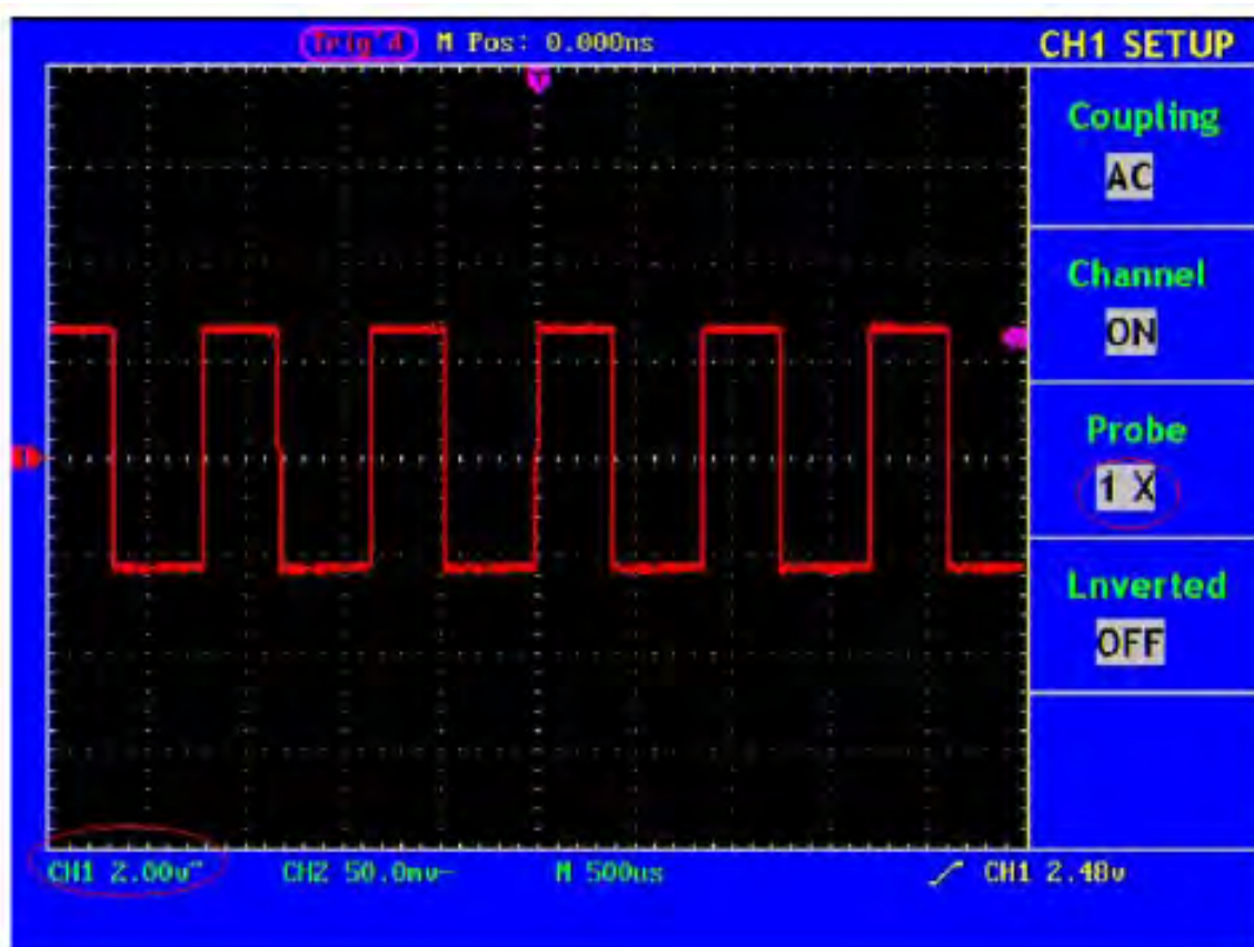
Abb. 17 Einstellen des Tastkopf-Dämpfungsfaktors
