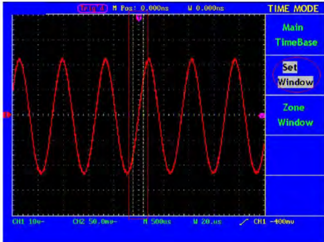
Abb. 24 Fenstereinstellung
