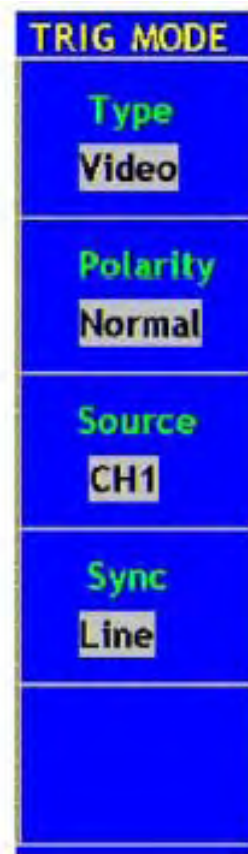
Abb. 30 Menü Video Trigger
