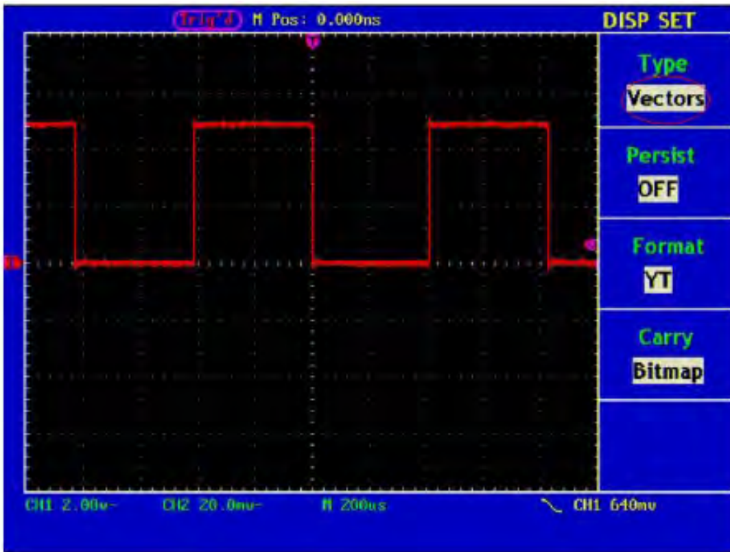
Abb. 38 Anzeige im Vektorformat
