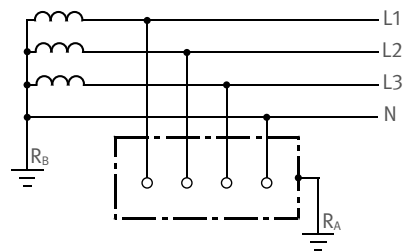
b) TT-System
