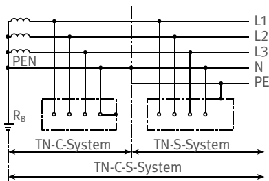
Abb. 3 Netzsystem
